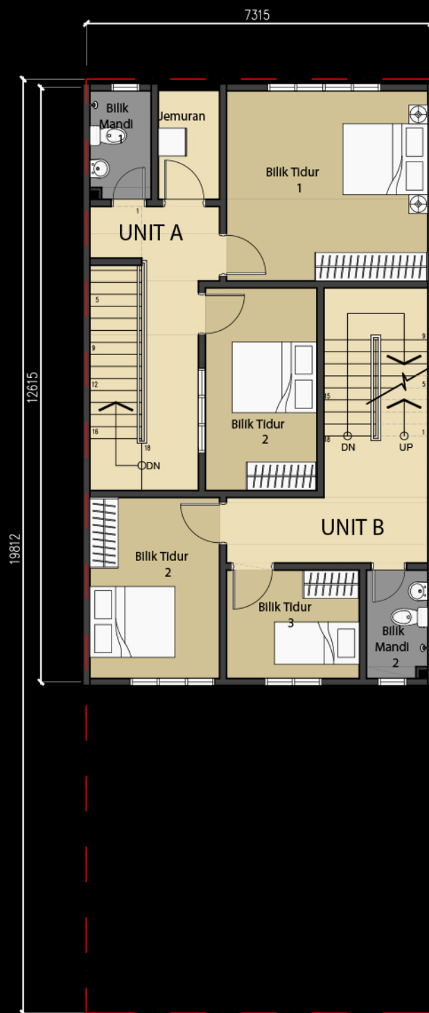
PELAN ARAS SATU
